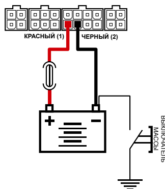
Подключение питания до выключателя массы
