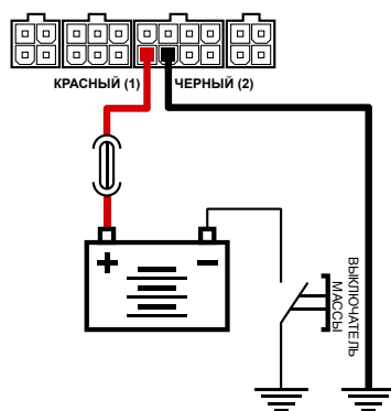
Подключение питания после выключателя массы
